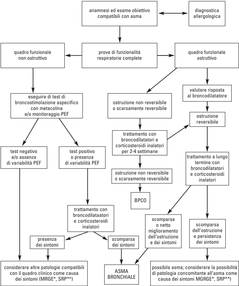
Figura 1.4 Algoritmo diagnostico
